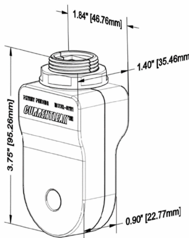
CT dimensions
